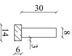
SZCZEGÓŁ OBRZEŻA 8x30x100
