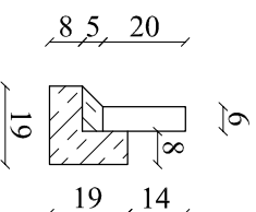
SZCZEGÓŁ OBRZEŻA NA ZIAZDACH
