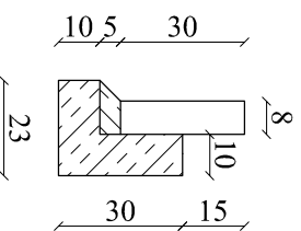
SZCZEGÓŁ OBRZEŻA 8x30x100
